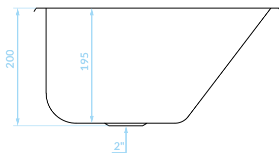
PRZEKRÓJ A-A
